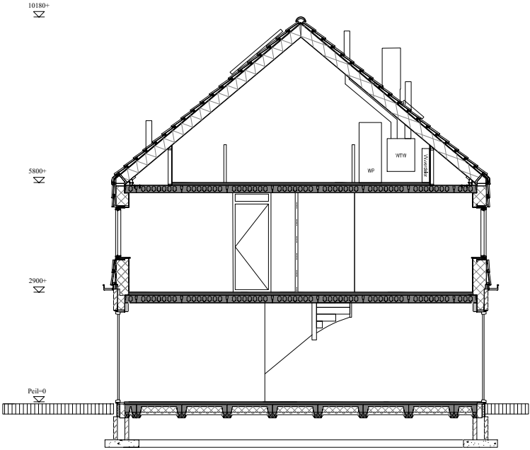
dwarsdoorsnede
