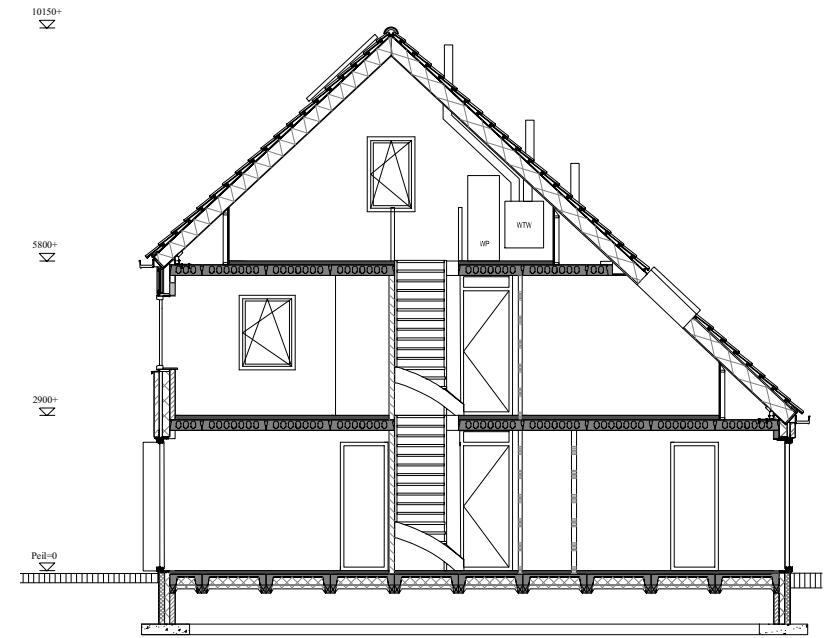
langsdoorsnede bnr: 3
