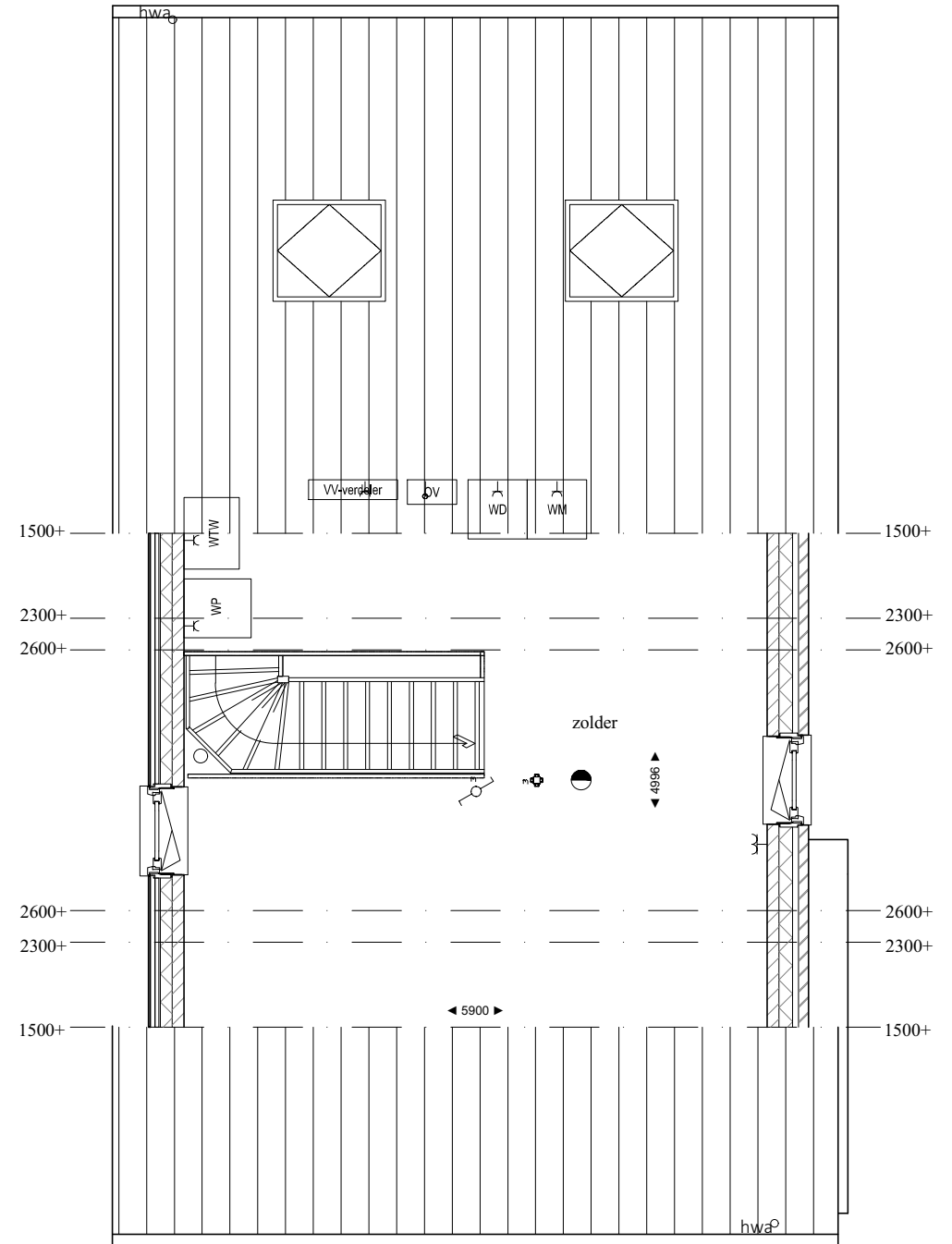
2e verdieping bnr: 4
