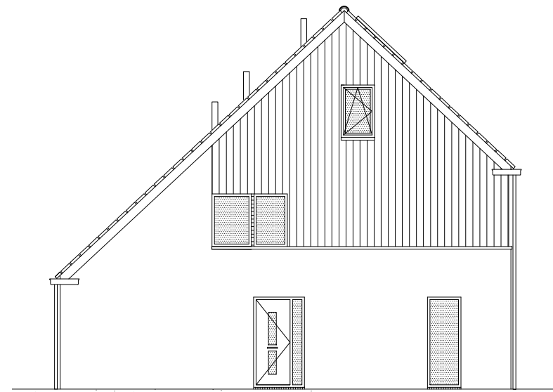
linker zijgevel bnr: 4
