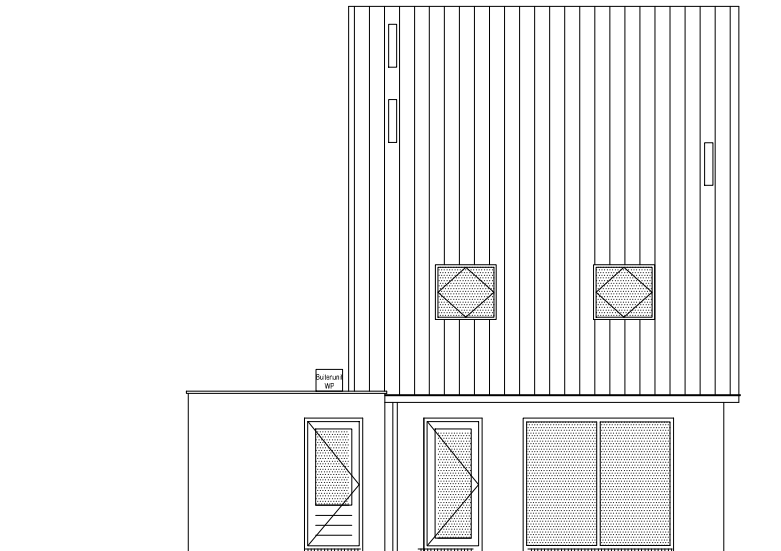
achtergevel bnr: 3
