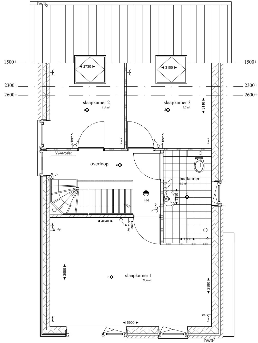
1e verdieping bnr: 4
