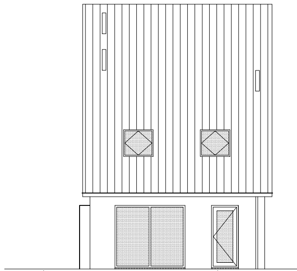
achtergevel bnr: 4
