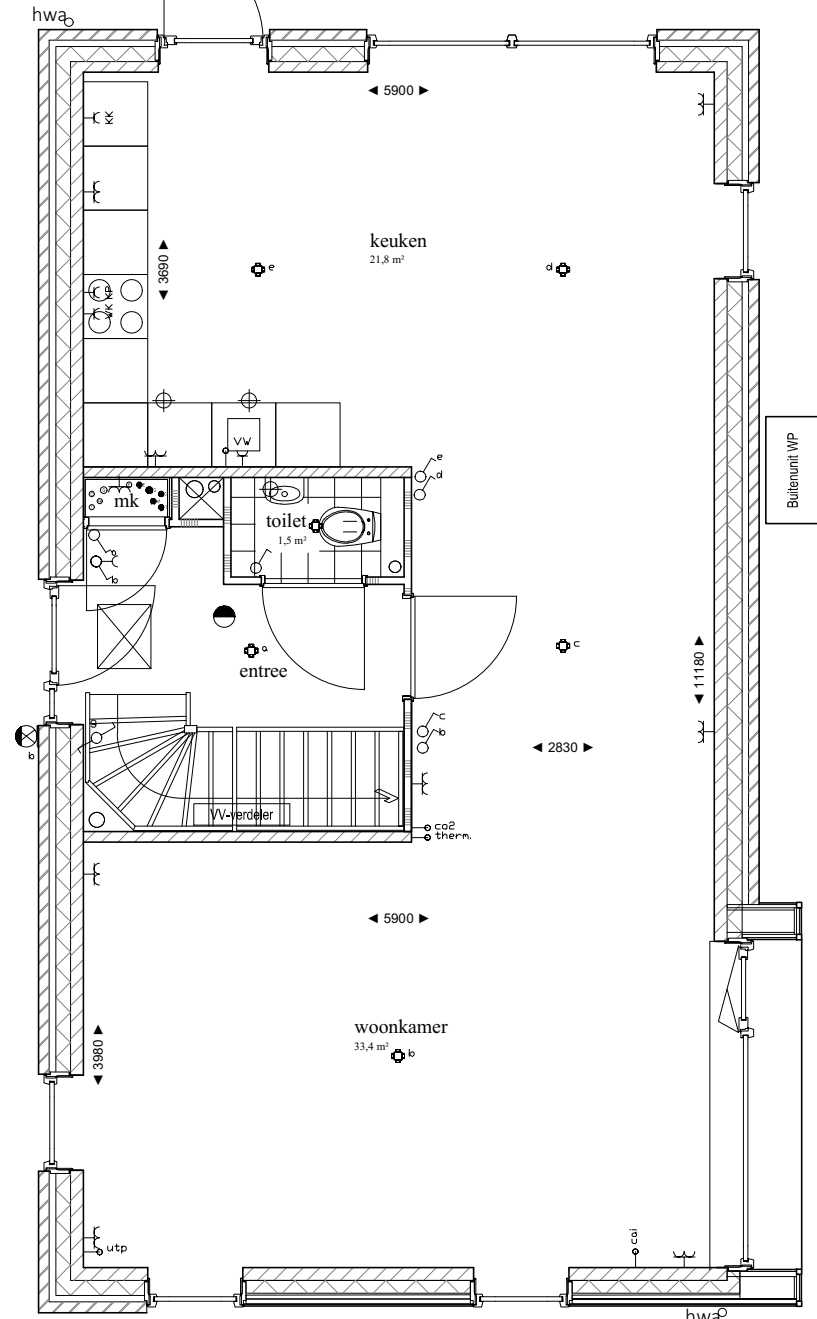
begane grond bnr: 4
