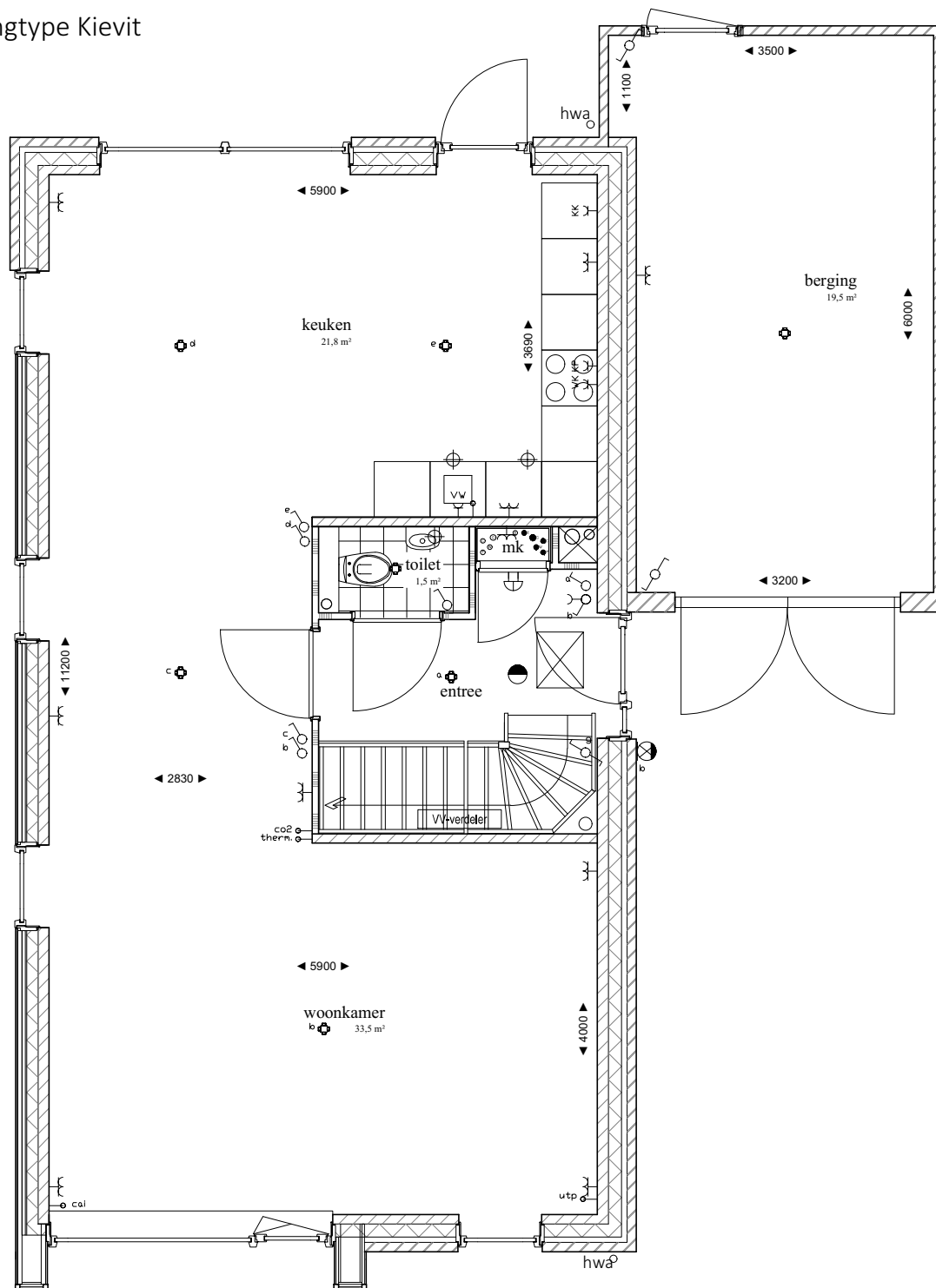
begane grond bnr: 3
