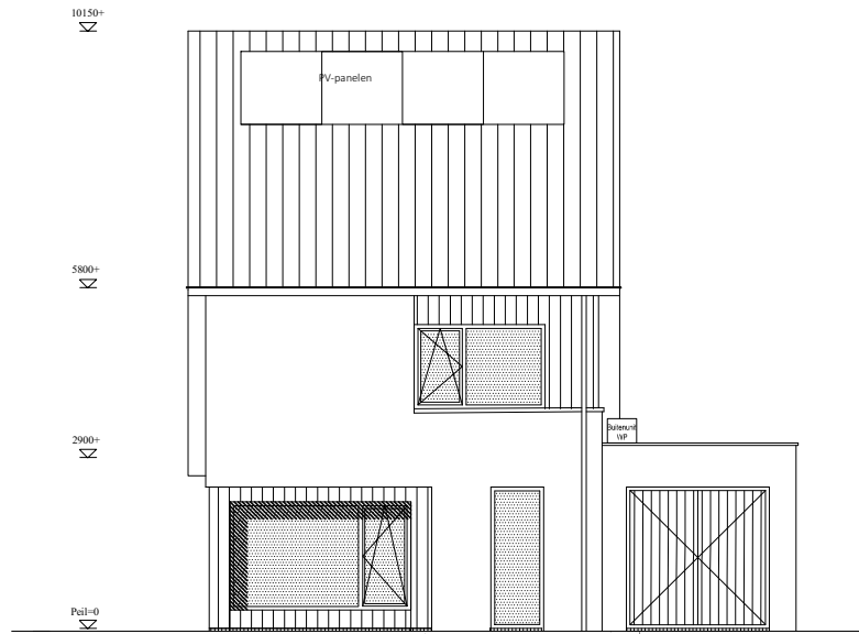
voorgevel bnr: 3
