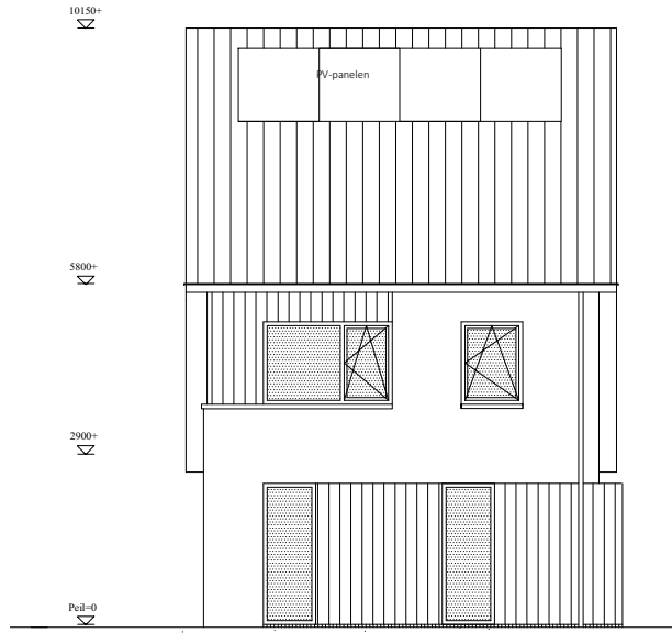
voorgevel bnr: 4
