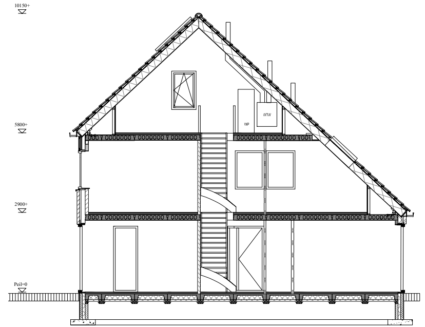
langs doorsnede bnr: 4
