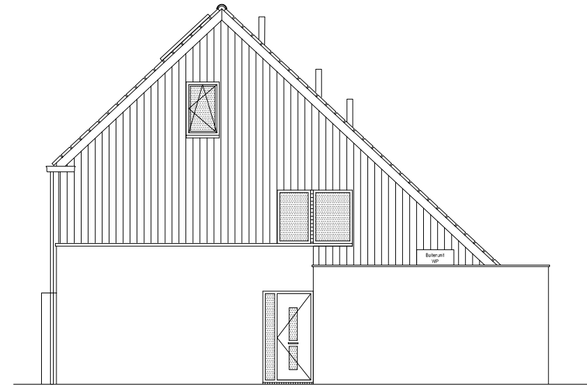
rechter zijgevel bnr: 3
