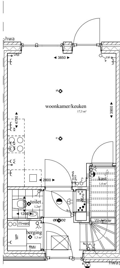
begane grond bnr: 10
