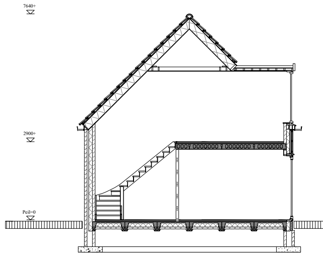
dwarsdoorsnede (2)
