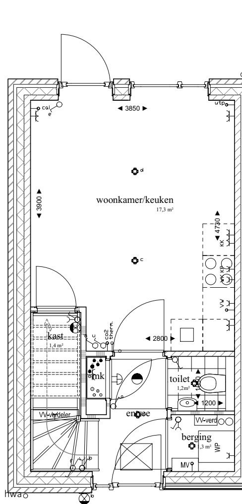
begane grond bnr: 9
