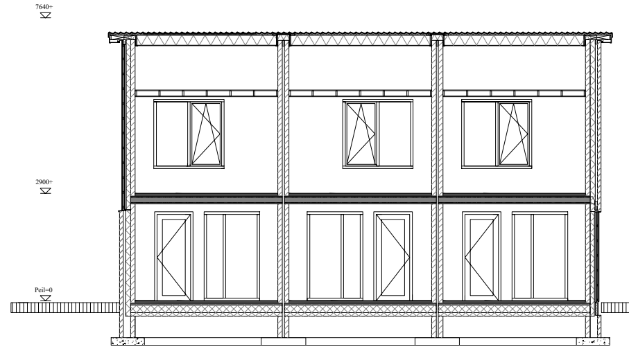
langsdoorsnede bnr: 9
