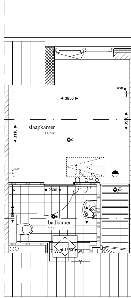
1e verdieping bnr: 10
