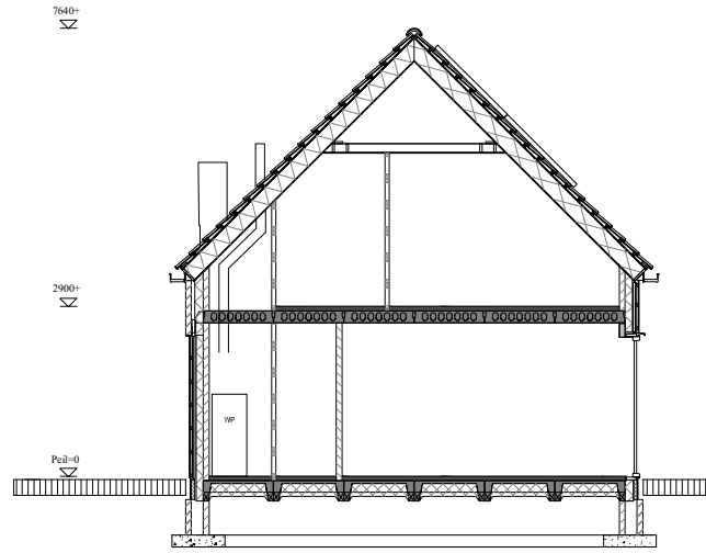
dwarsdoorsnede
