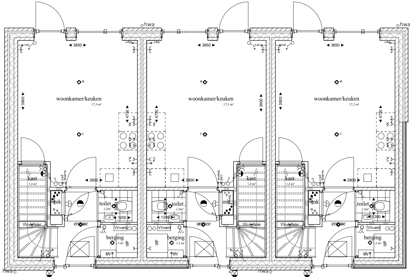
begane grond bnr: 9
